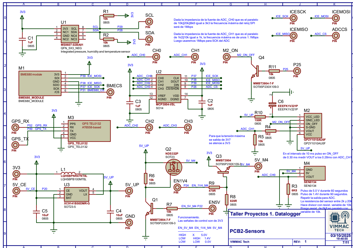
Ilustración 7: PCB 2 esquemático 1
