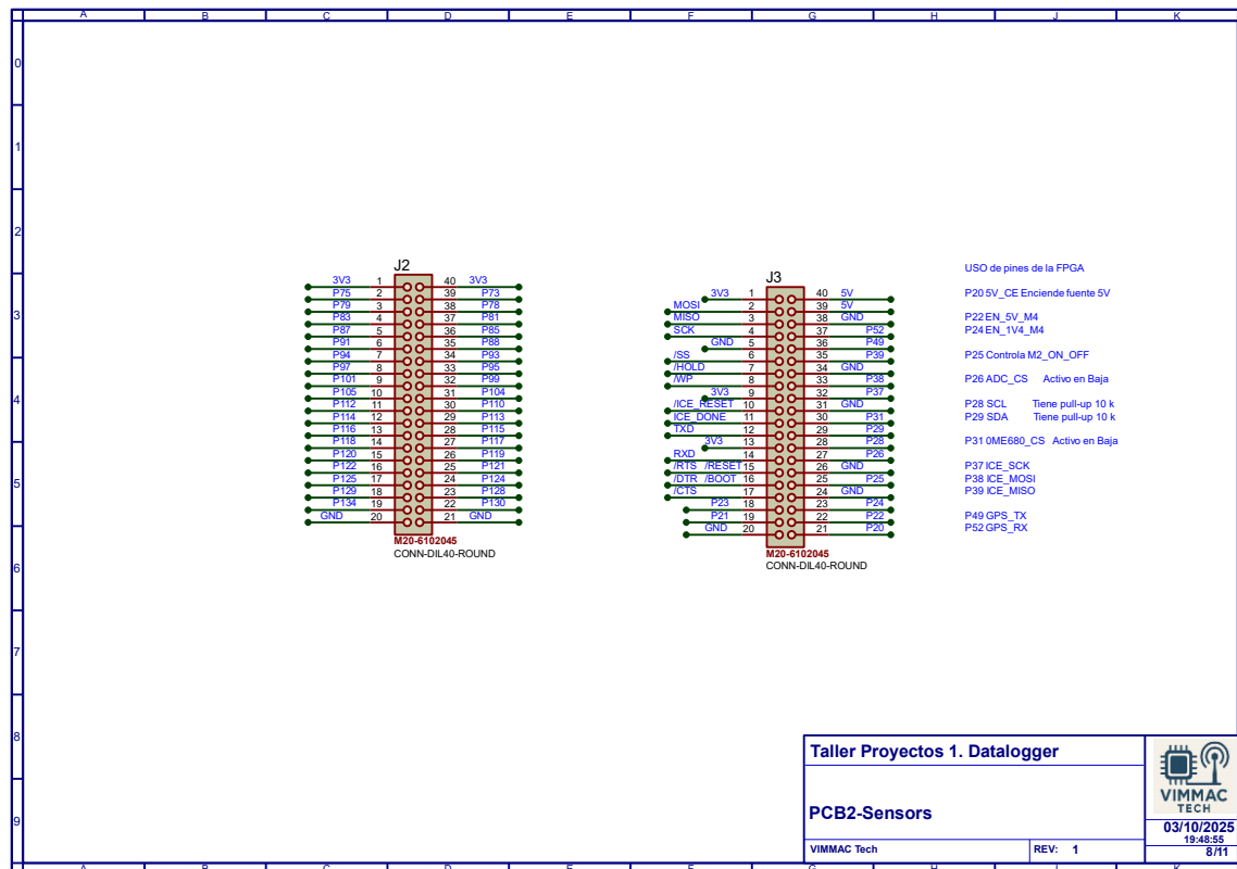
Ilustración 8: PCB2 esquemático 2
