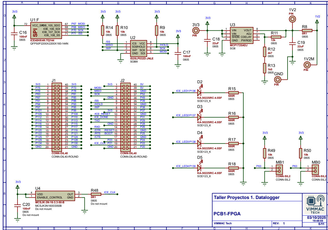
Ilustración 5: PCB1 esquemático 2
