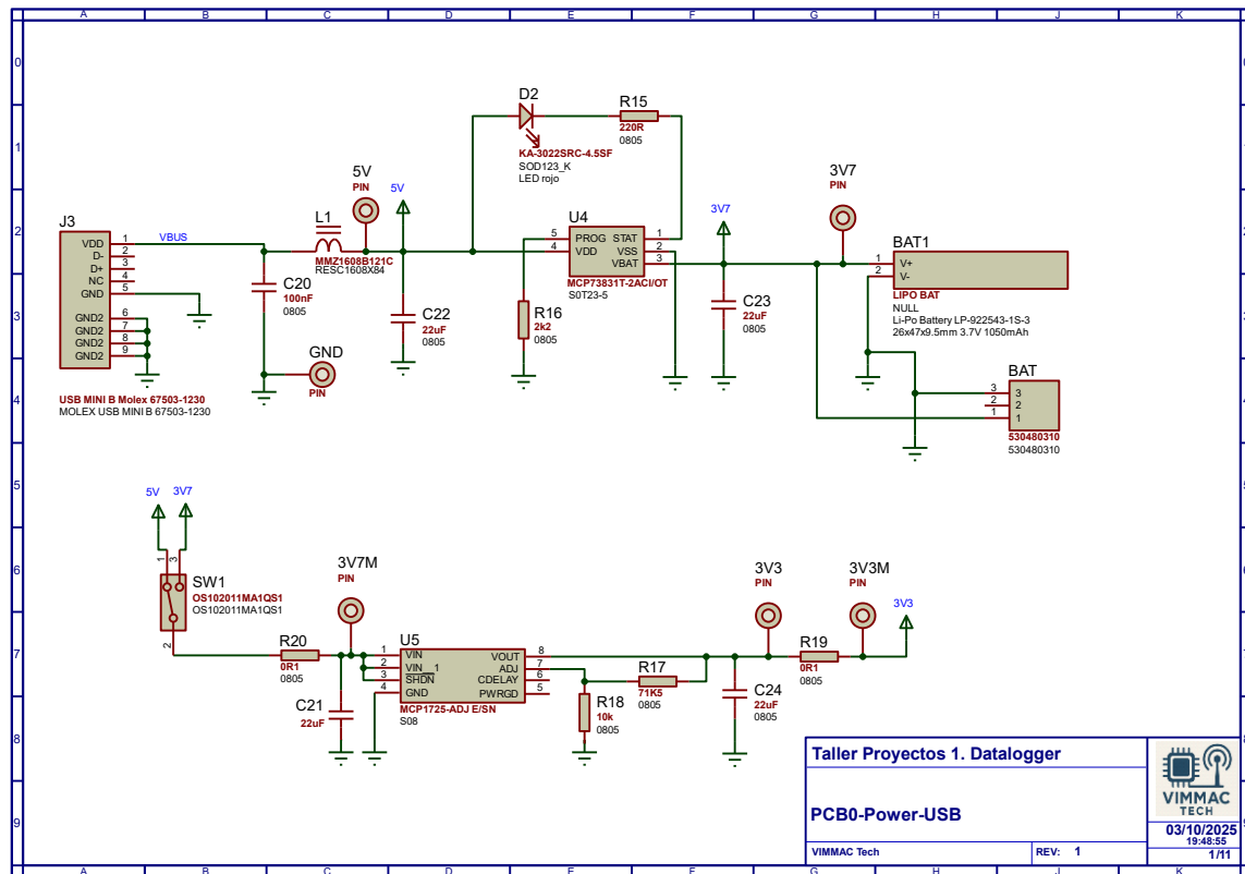
Ilustración 1:PCB 0 esquemático 1
