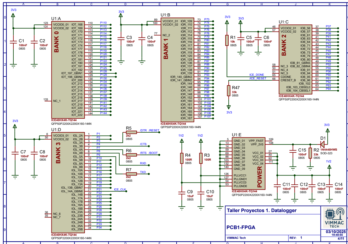
Ilustración 4: PCB1 esquemático 1
