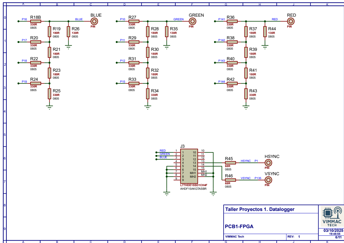
Ilustración 6: PCB1 esquemático 3
