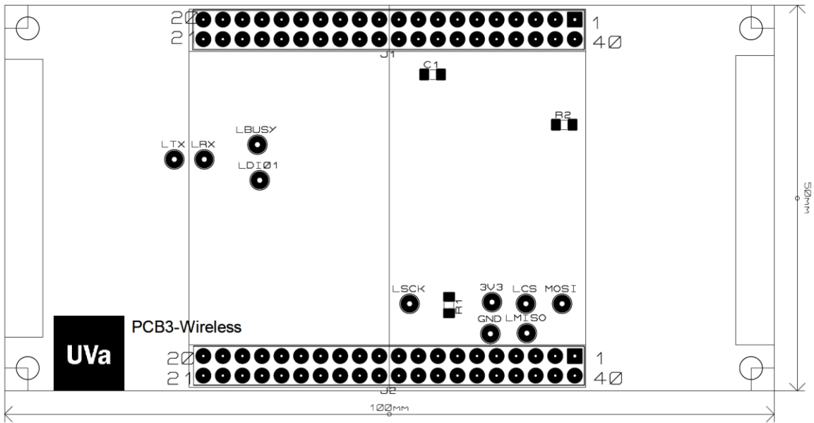
Ilustración 2: PCB3
