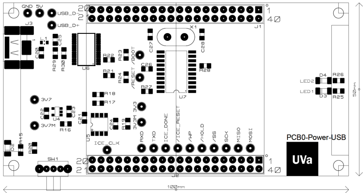
Ilustración 1: PCB 0
