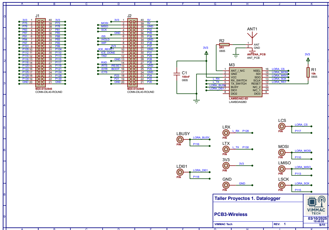
Ilustración 9: PCB esquemático 1
