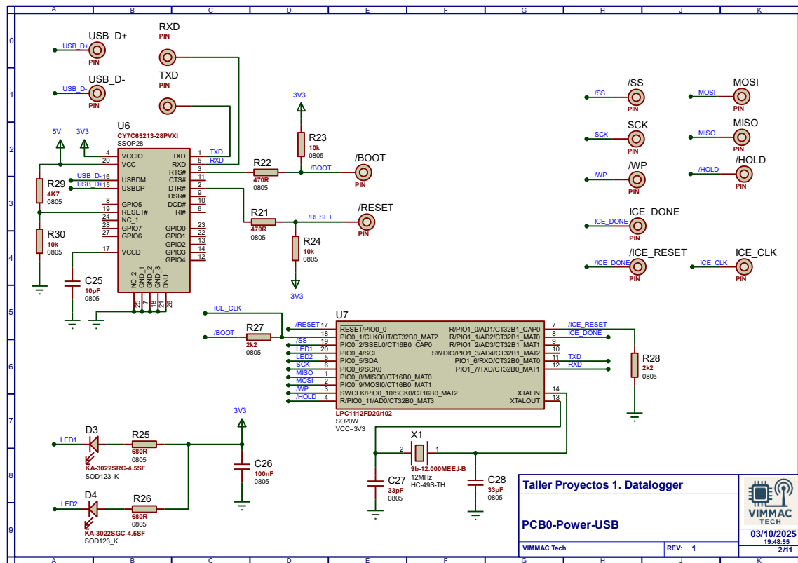
Ilustración 2: PCB 0 esquemático 2
