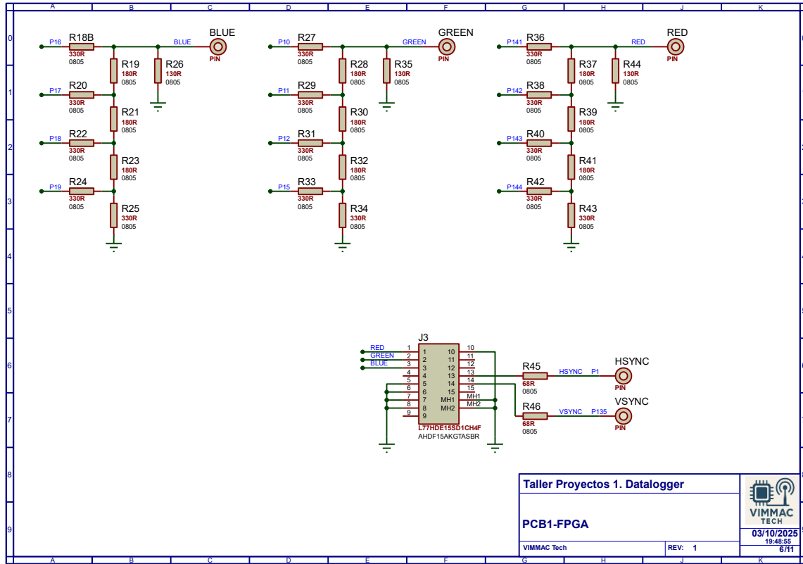
Ilustración 6: PCB1 esquemático 3
