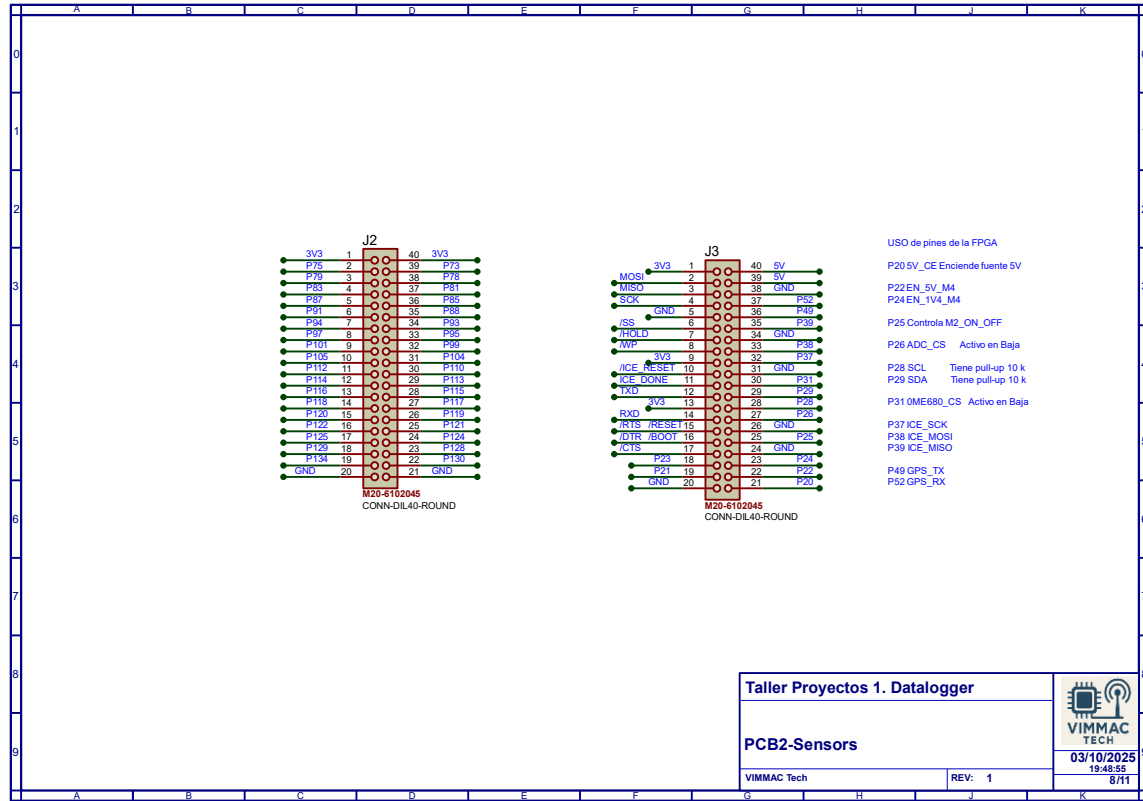
Ilustración 8: PCB2 esquemático 2
