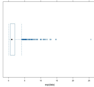
(d) Boxplot
