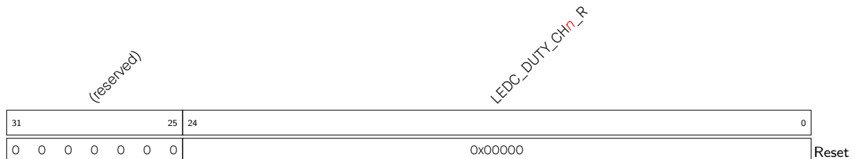
Register 53.12. LEDC_CH n _DUTY_R_REG ( n : 0-7) (0x0010+0x14* n )
