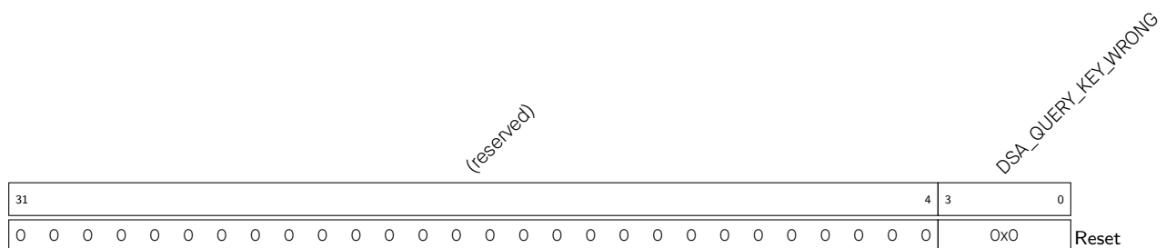
Register 29.6. DSA_QUERY_KEY_WRONG_REG (0x0E10)
