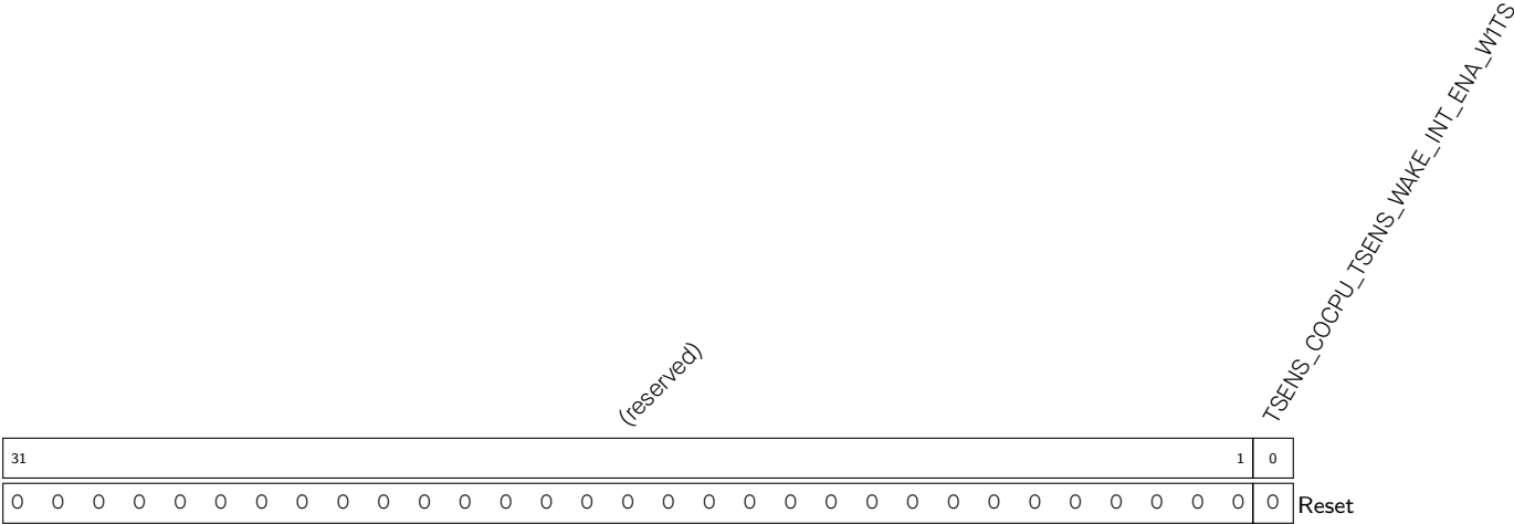
Register 59.7. TSENS_INT_ENA_WITS_REG (0x001C)
