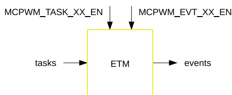
Figure 54.3-4. ETM Module
