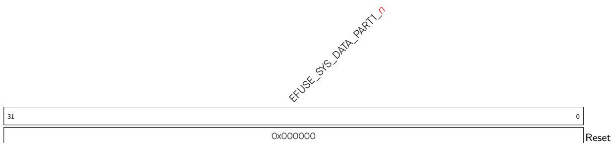
Register 8.15. EFUSE_RD_SYS_PART1_DATA n _REG ( n : 0-7) (0x005C+0x4* n )
