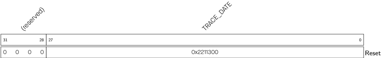
Register 2.19. TRACE_DATE_REG (0x03FC)
