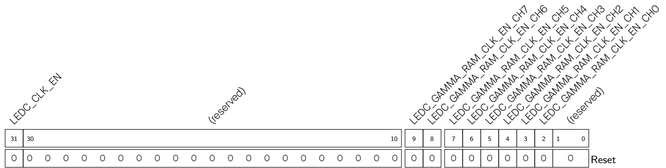
Register 53.11. LEDC_CONF_REG (0x0170)
