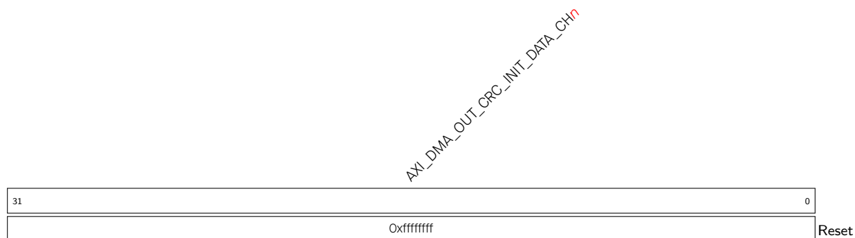
Register 4.91. AXI_DMA_OUT_CRC_INIT_DATA_CH n _REG ( n : 0-2) (0x0180+0x68* n )
