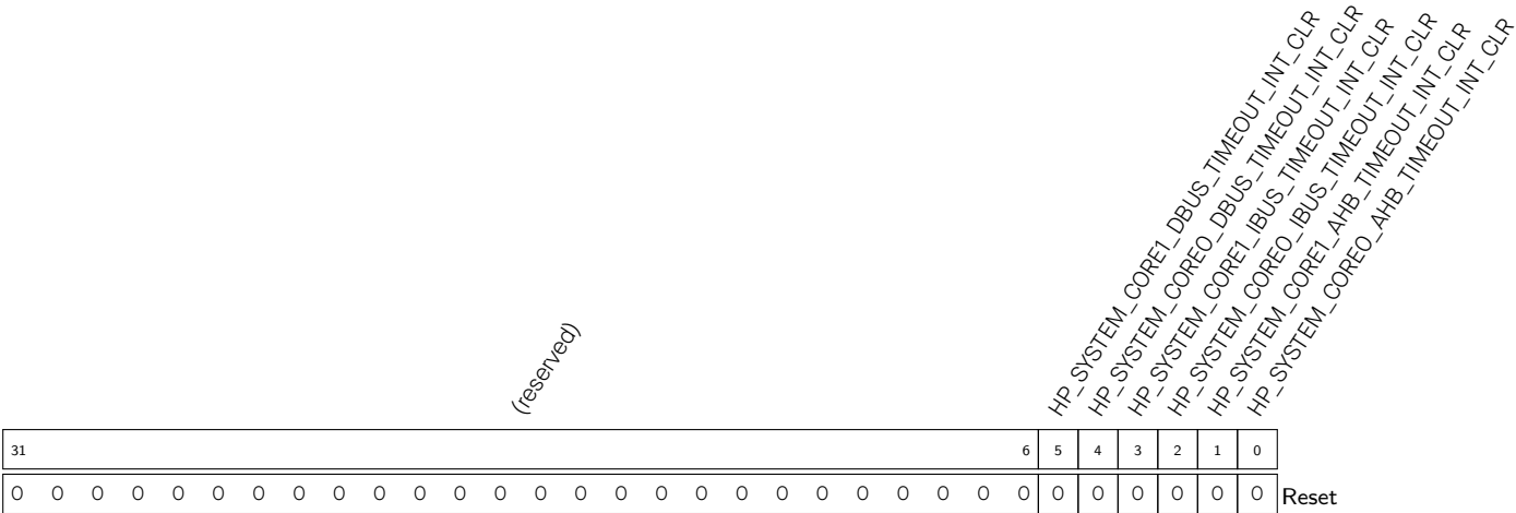
Register 20.14. HP_SYSTEM_HP_CORE_TIMEOUT_INT_CLR_REG (0x01B4)
