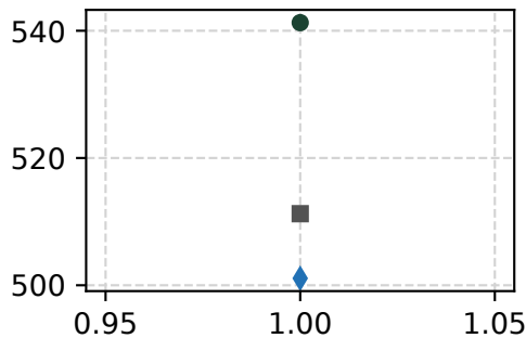
(b) ShareGPT
