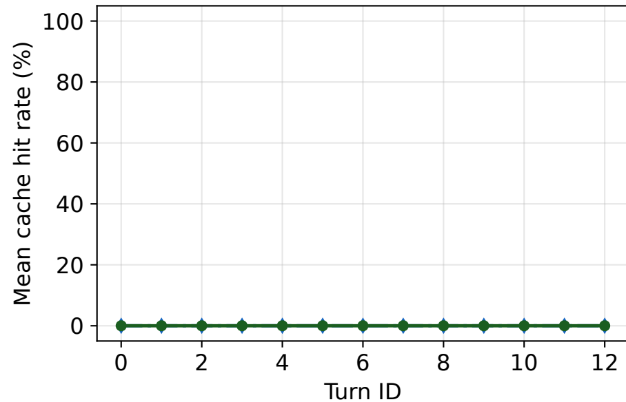
LMSys-Chat
