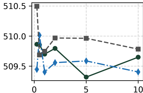
(b) ShareGPT
