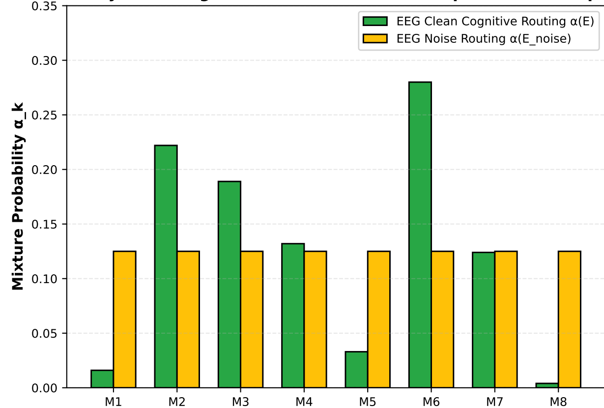
(d) Dynamic Cognitive Allocation Across 8 Spatial Basis Maps
