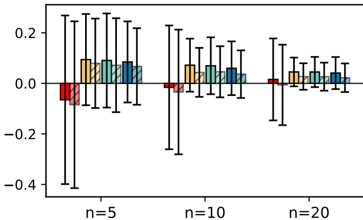
Density (D)
