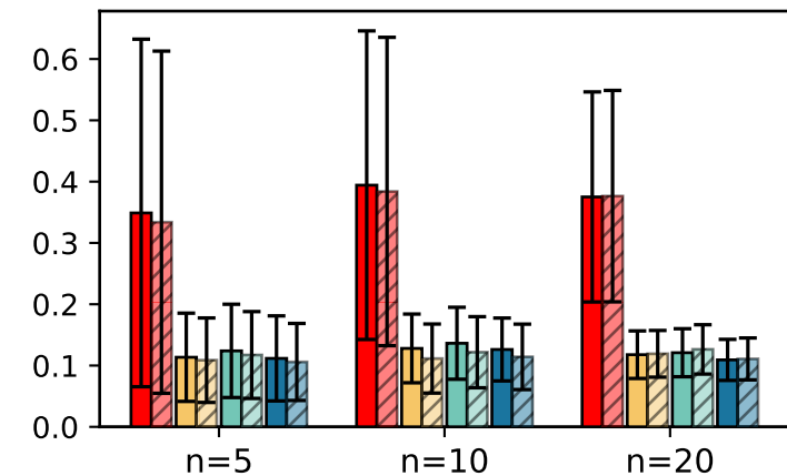
Voronoi (V)
