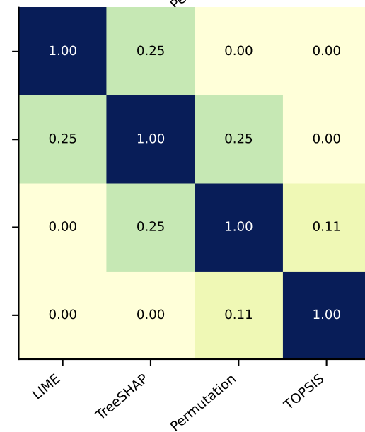
Jaccard@5
