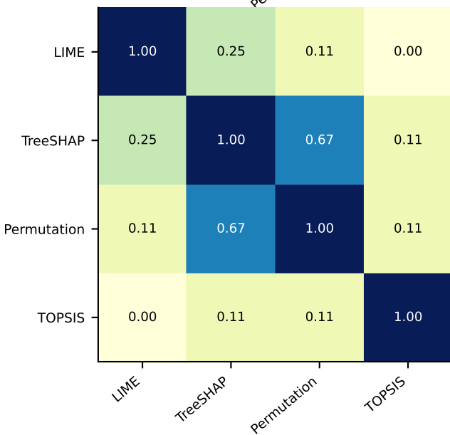
Jaccard@5
