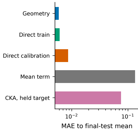
(d) Direct-risk baselines
