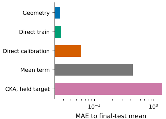
(d) Direct-risk baselines
