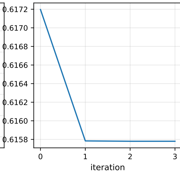
IRLS / Newton (quadratic)
