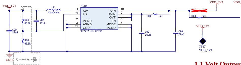
1.1 Volt Output
