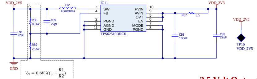
2.5 Volt Output
