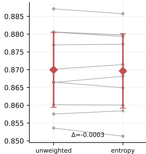
MaxEnt
