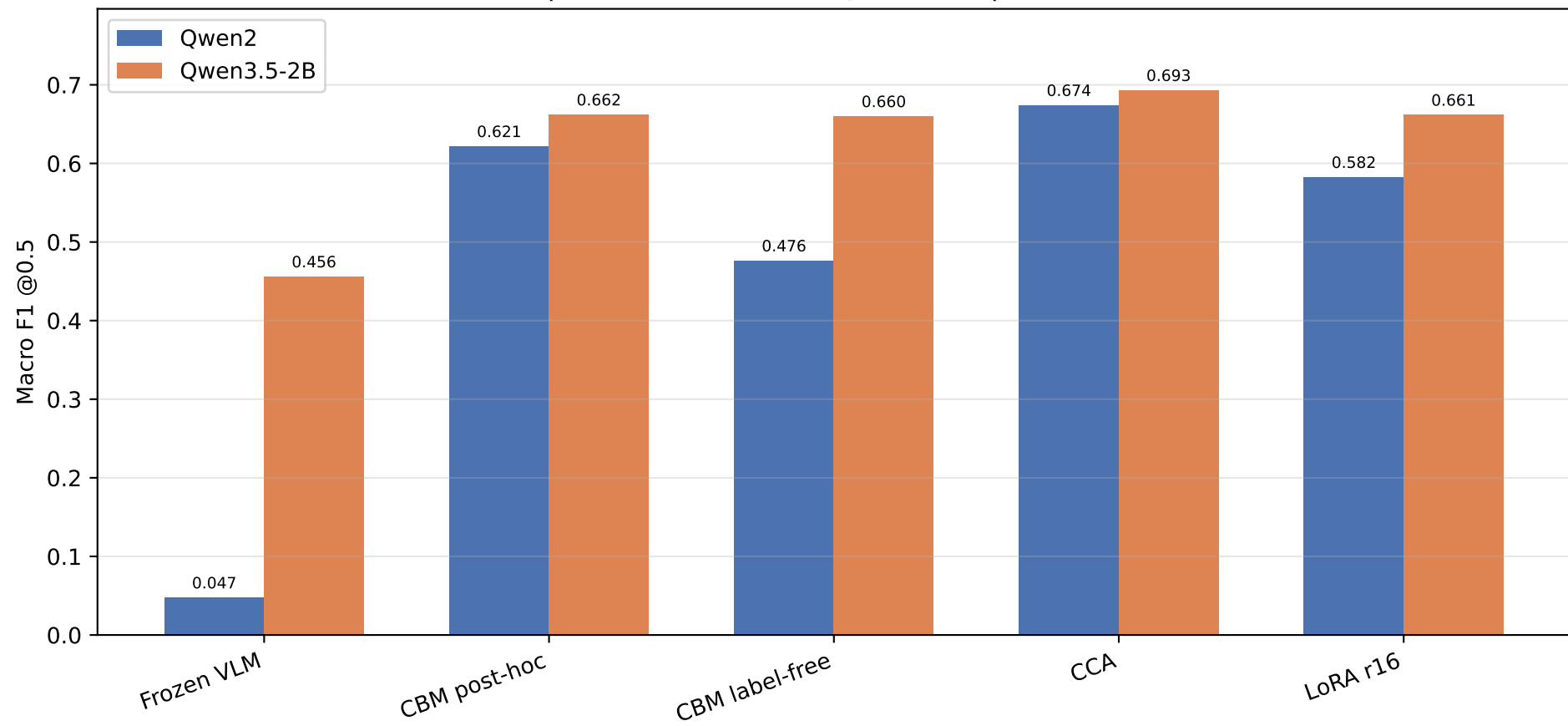
CheXpert test — Macro F1 @0.5 (fair splits, n=9,197)
