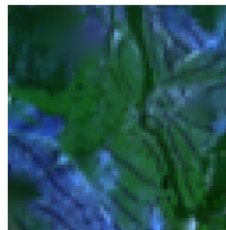
exemplar_based
