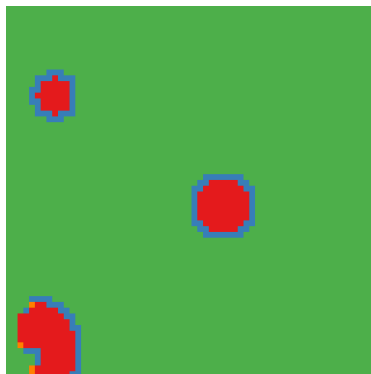
bicubic (LISA)
