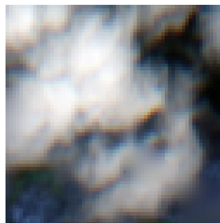
kriging
