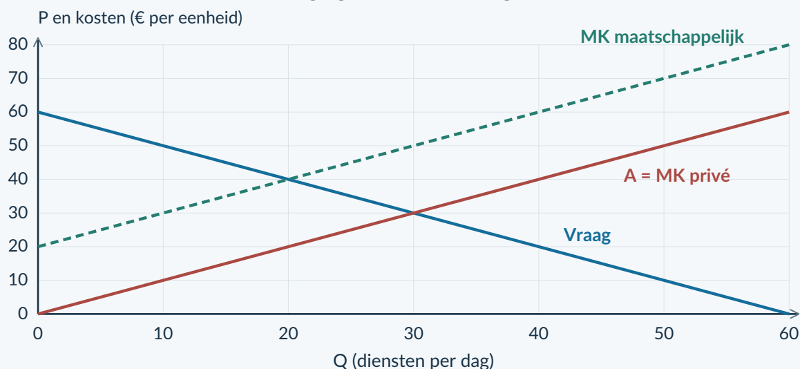
Figuur 20. De private en maatschappelijke kosten zijn gegeven. Voeg de uitkomsten en het gevraagde verliesgebied toe.
