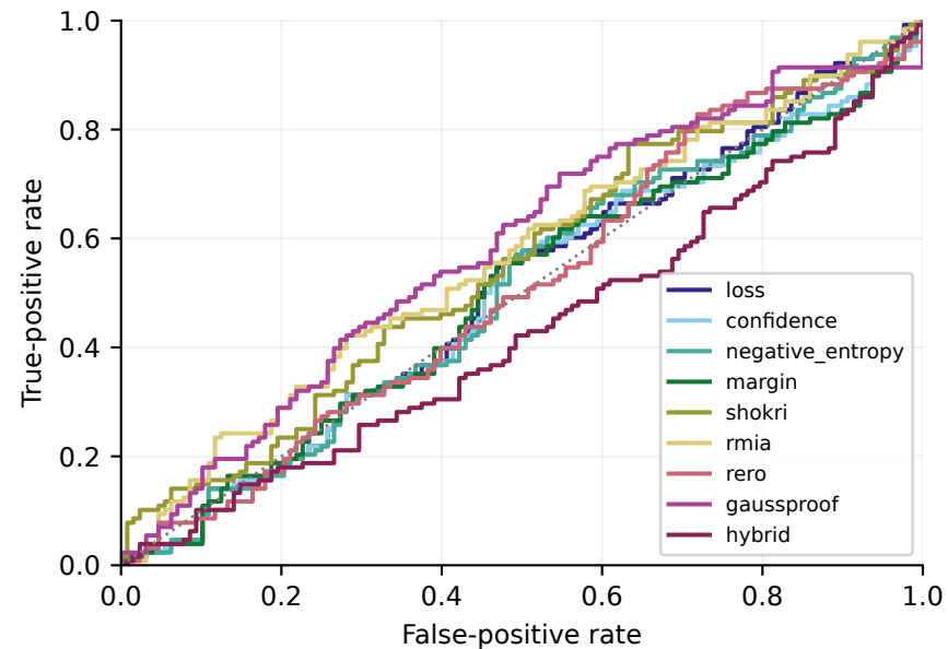
seed17_sigma0_clip1_B32
