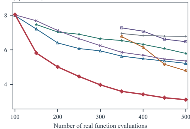
(d) WFG7, M = 10
