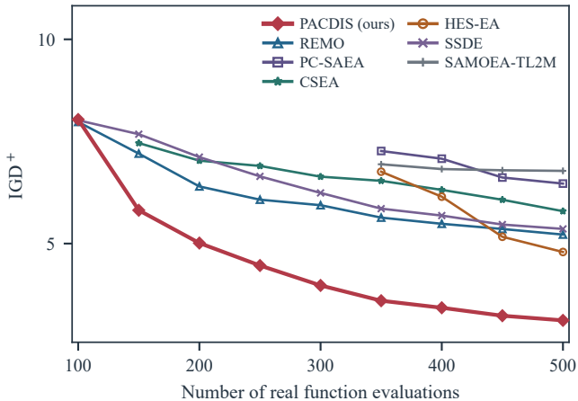
(d) WFG7, M = 10
