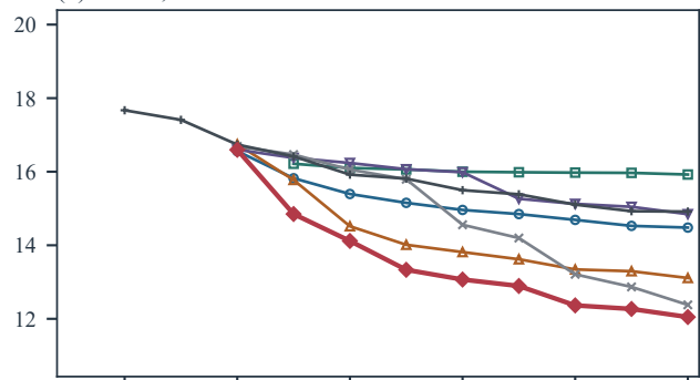
(d) WFG8, M = 15
