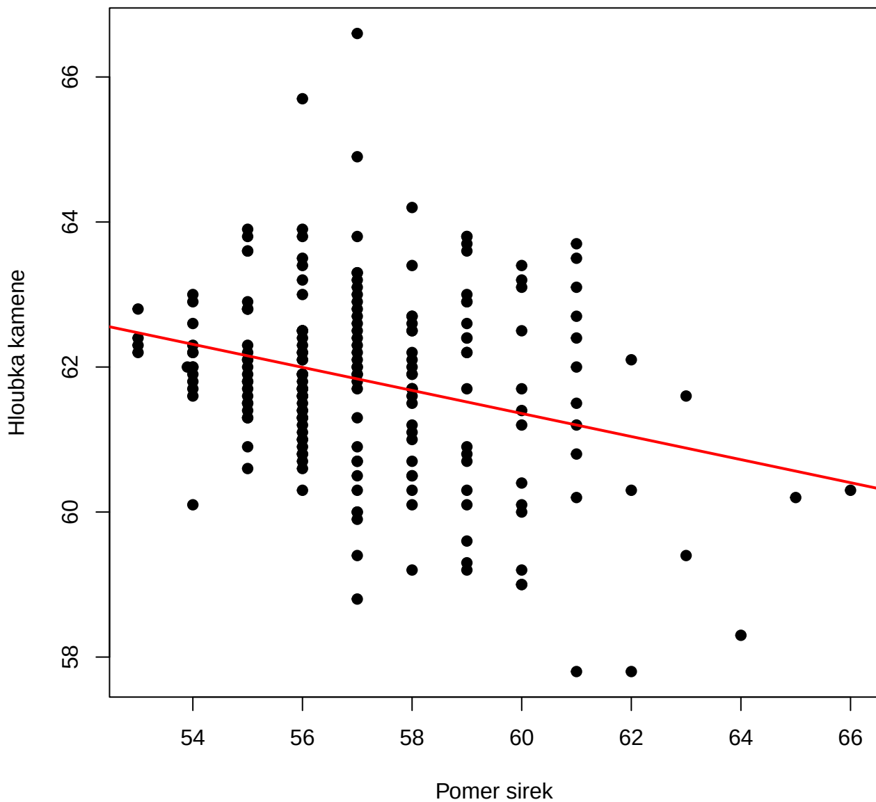
Rozptylový graf
