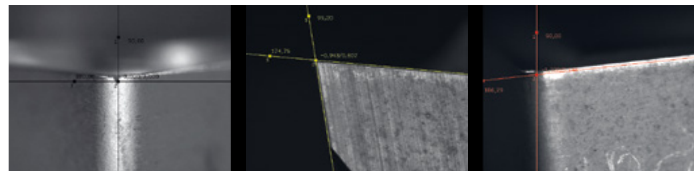
Festes Fadenkreuz zum Einstellen und Messen der Spitzenhöhe.
