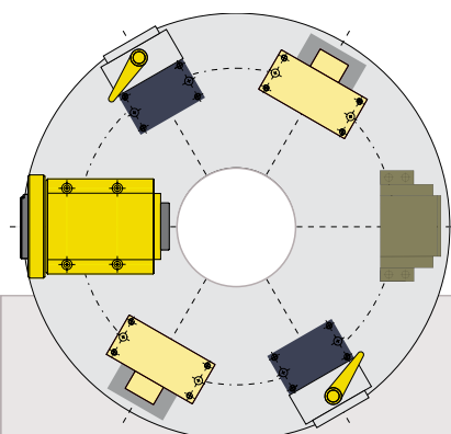
Bestückung D 745 – 6-fach Teilung
