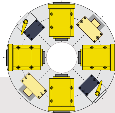
Bestückung D 745 – 8-fach Teilung
