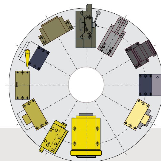
Bestückung D 900 – 12-fach Teilung
