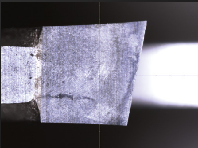
Radiale Ansicht Sägeblattzahn zur Kontrolle Schneide und Einlötlung
