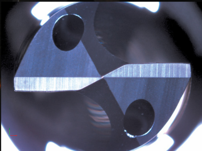
Stirransicht Stufenbohrer im »pomLightTube«
