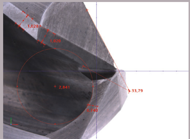
Konturmessung im »pomLightTube«
