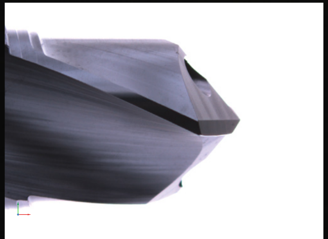
Umfangsansicht Stufenbohrer im »pomLightTube«
