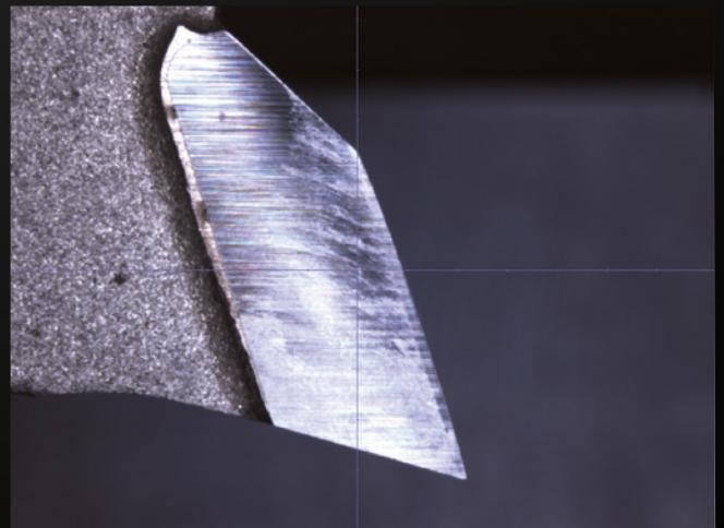
Axiale Ansicht Sägeblattzahn zur Kontrolle Schneide und Einlötlung
