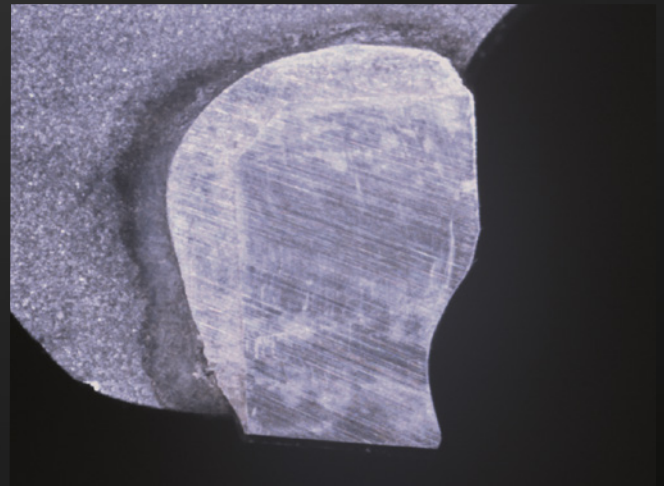
Axiale Ansicht Sägeblattzahn mit Spanleitstufe
