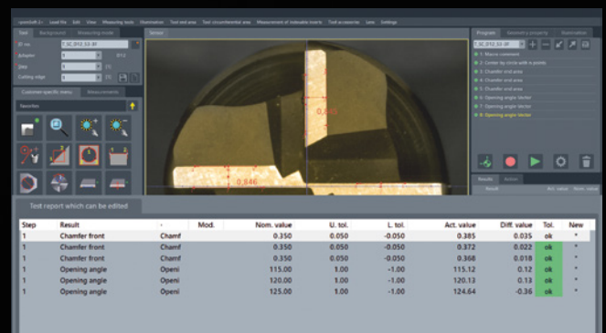
Übersicht aller ermittelten Messergebnisse mit Toleranzen
