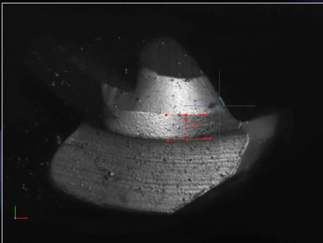
Inspektion an einem Vollradiusfräser D 0,2 mm
