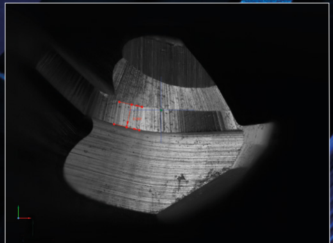
Inspektion an einem Vollradiusfräser D 0,6 mm
