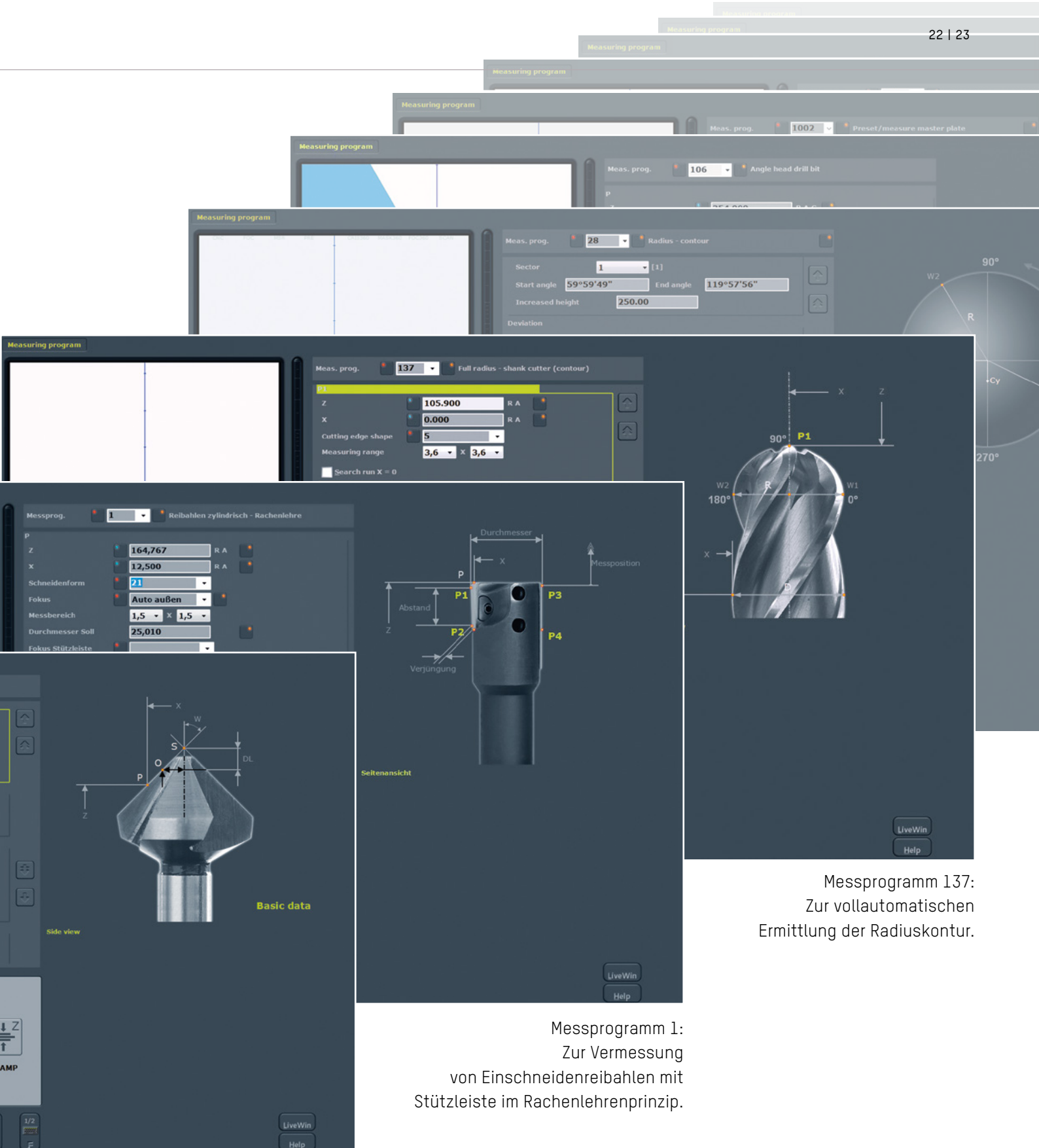
Messprogramm 17: Zur Ermittlung der theoretischen Spitze über Schneidenform.
