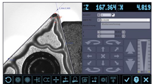
»metis« Werkzeuganalyse
