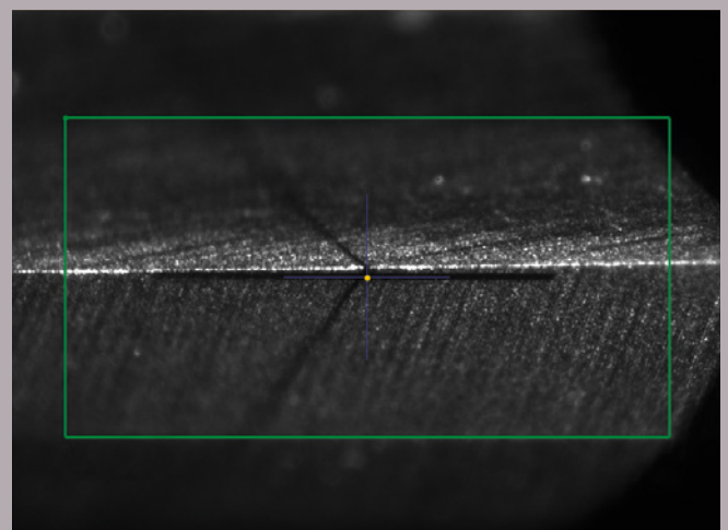
Messung Schneidkantenpräparation mit »zep«-Sensor
