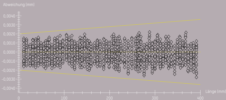
Zweidimensional – in Anlehnung an die DIN EN ISO 10360, E_{xy} = 2,0 \mu\text{m} + (L/250 \text{ mm}) \mu\text{m}
