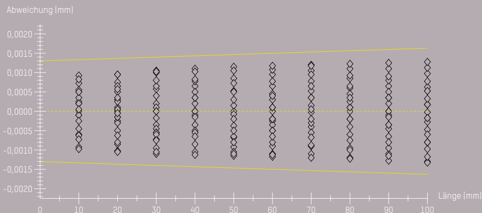
Eindimensional – nach VDI/VDE 2617, E_x = 1,3 \mu\text{m} + (L/300 \text{ mm}) \mu\text{m}
