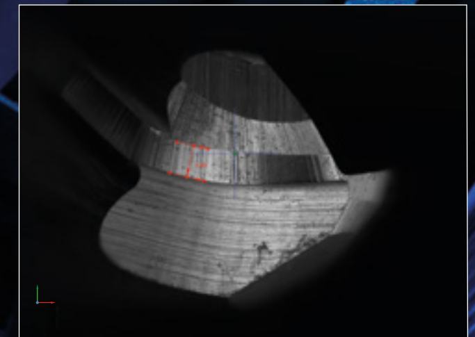
Inspektion an einem Vollradiusfräser D 0,6 mm
