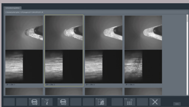
Messprogramm 482 – Übersicht der aufgenommenen Schneidenbilder inklusive Messfunktion zur Verschleißbestimmung.
