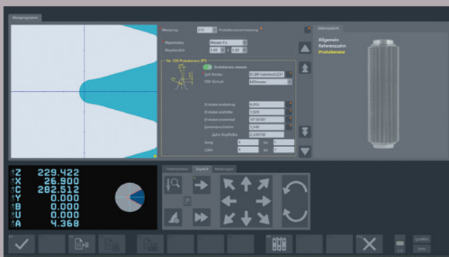
Messprogramm 315 – Datenanlage im fotorealen Eingabediaglog »fored«.
