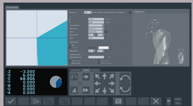
Spitzenwinkel mit Hohlsliff – wird an Bohrwerkzeugen sowie an hohlgeschliffenen Werkzeugschneiden vom Startpunkt (Außendurchmesser) bis zur Werkzeugspitze oder dem definierten Endpunkt durch Konturverfolgung ermittelt.
