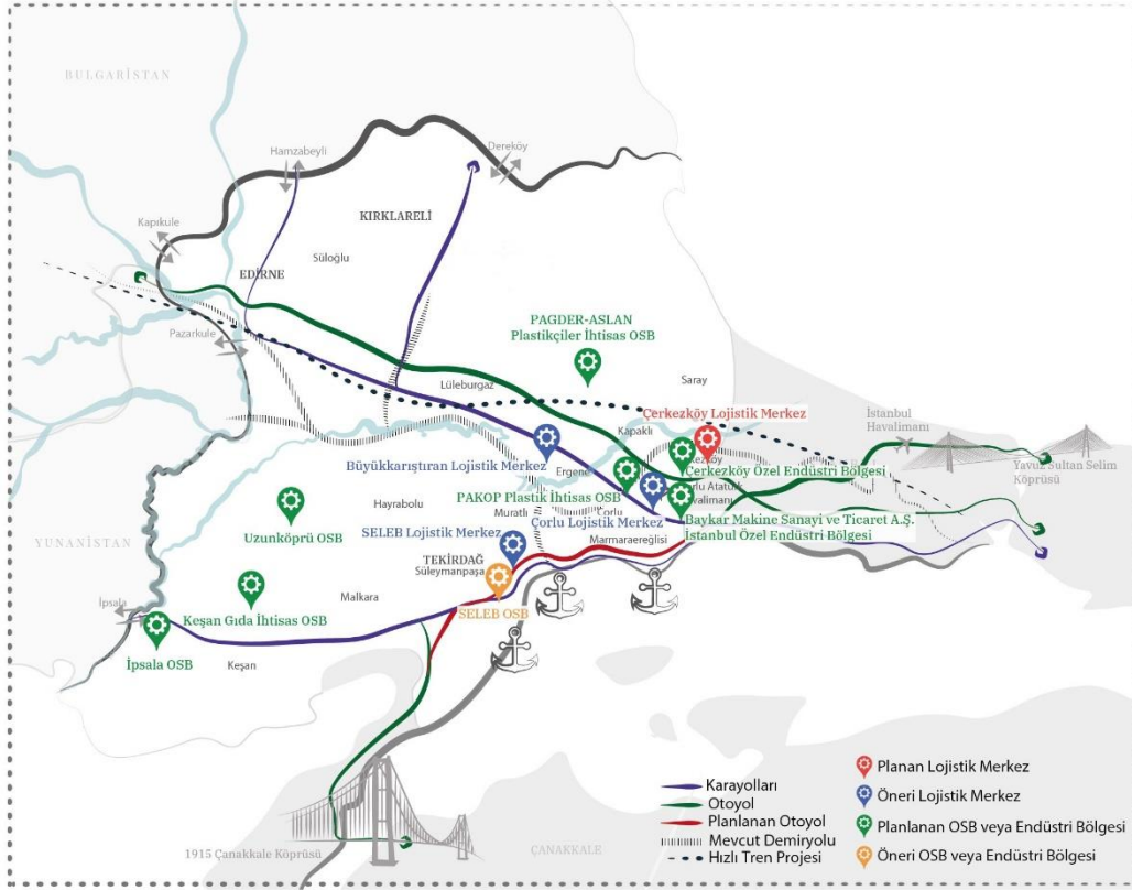
Şekil 18: Planlanan ve Öneri Organize Sanayi Bölgeleri, Endüstri Bölgeleri ve Lojistik Merkezler
