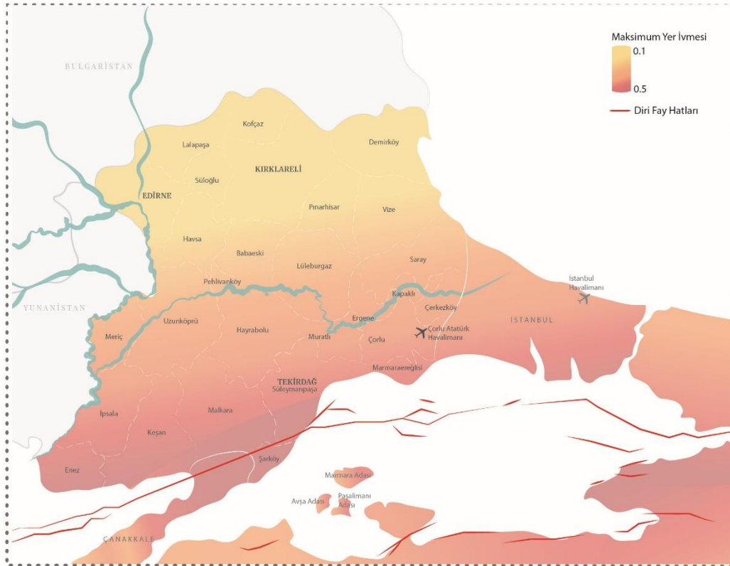
Şekil 24: Diri Fay Hatları ve Bölge Deprem Tehlike Haritası
