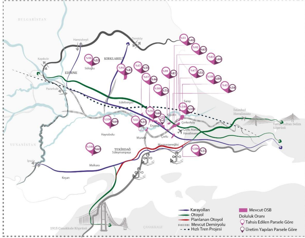
Şekil 17: Mevcut Organize Sanayi Bölgeleri ve Endüstri Bölgeleri
