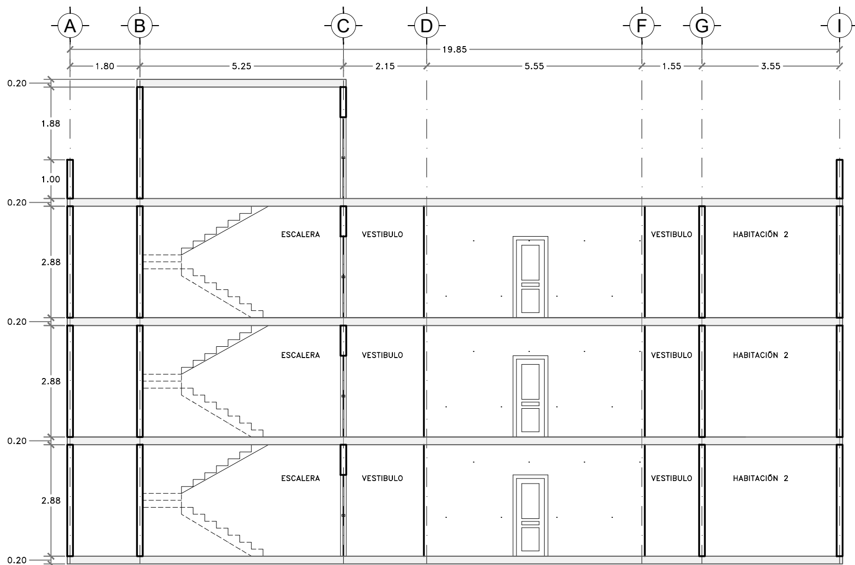
CORTE A-A' ESC 1:100 200 000 M2
