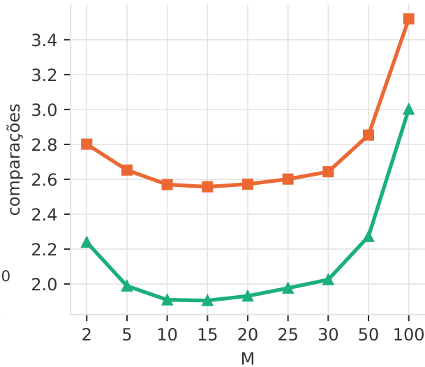
1e6 Comparações (n = 100.000)
