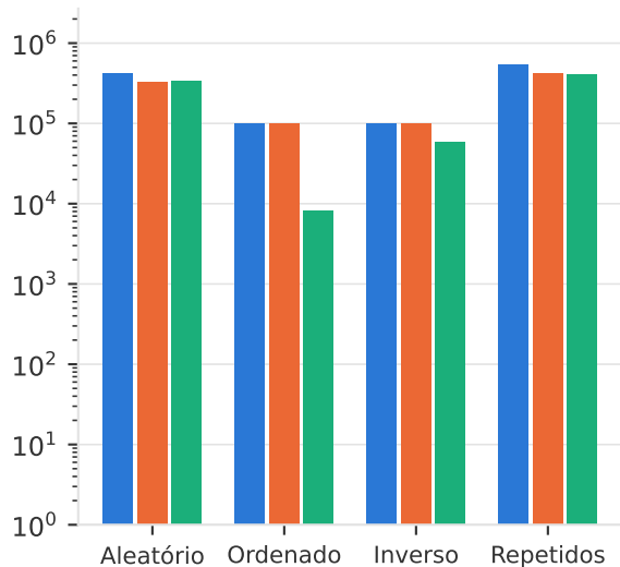
Trocas (n = 100.000)
