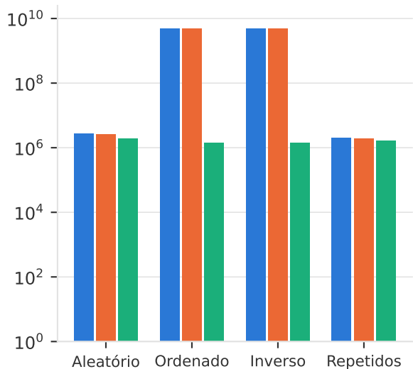
Comparações (n = 100.000)
