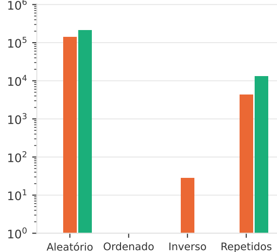
Deslocamentos (n = 100.000)
