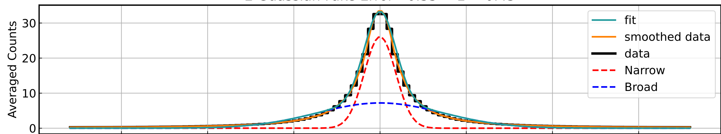
2 Guassian Fake Error - 0.35 < z < 0.45
