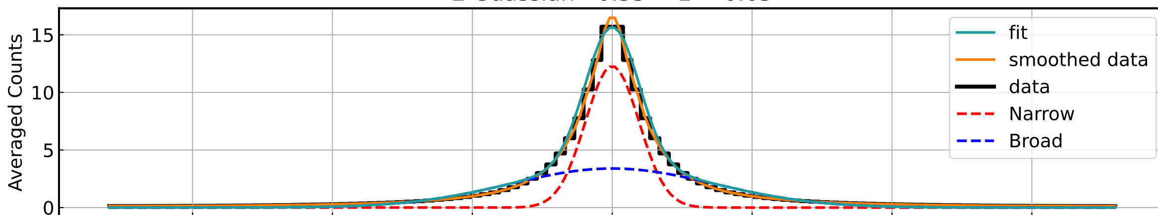
2 Guassian - 0.55 < z < 0.65
