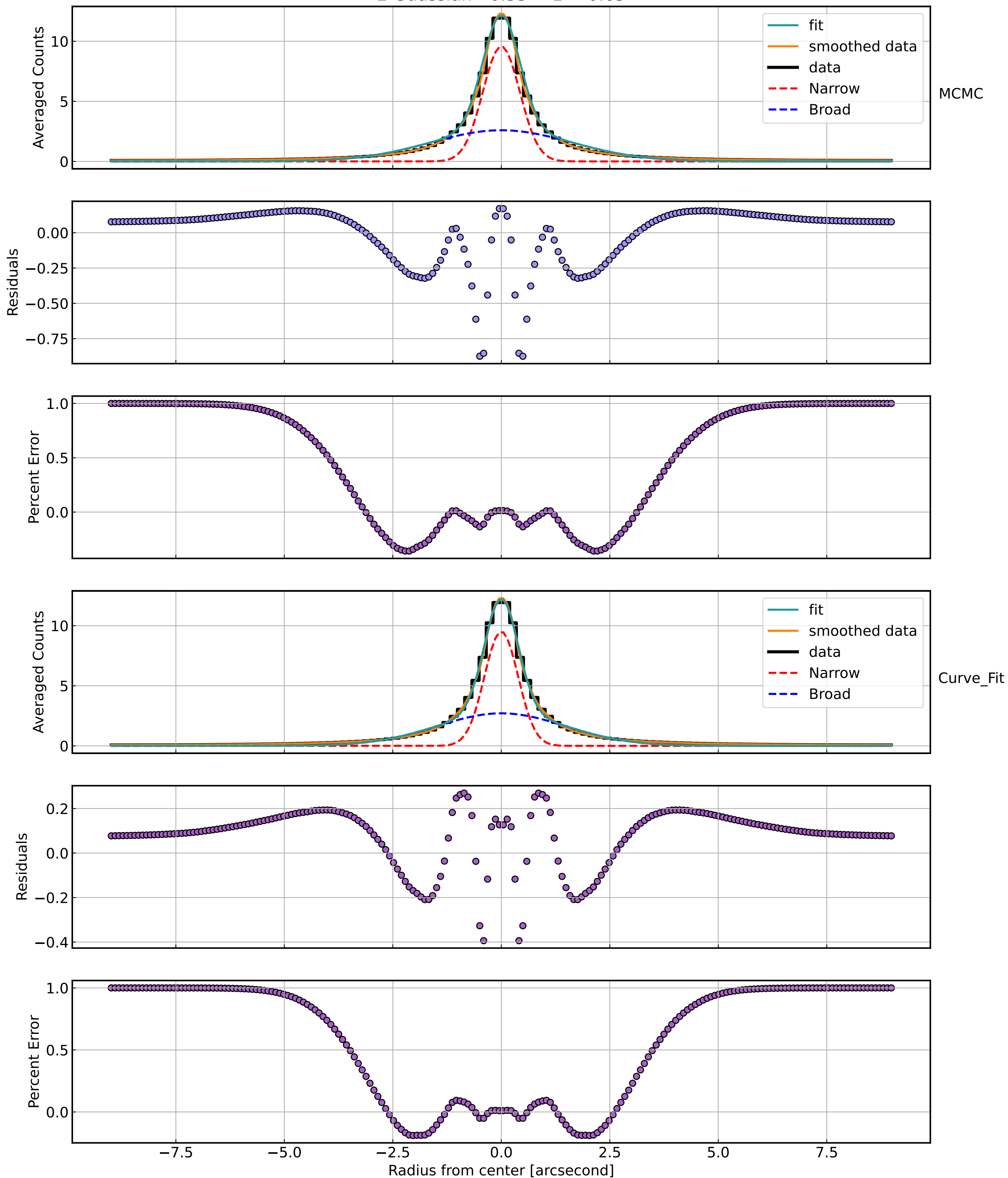
2 Guassian - 0.55 < z < 0.65
