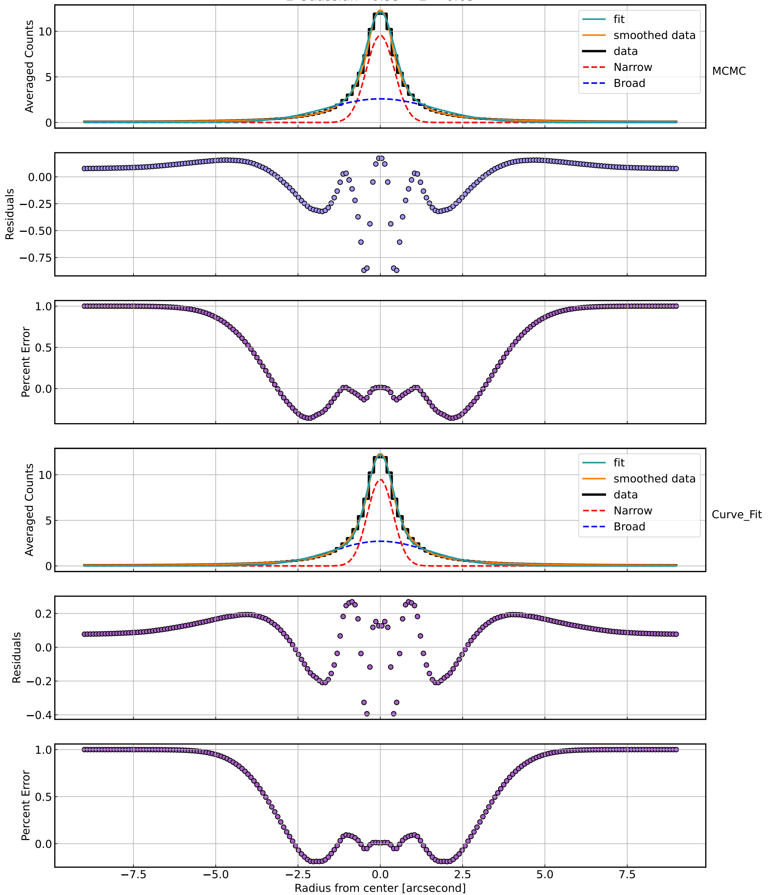
2 Guassian - 0.55 < z < 0.65
