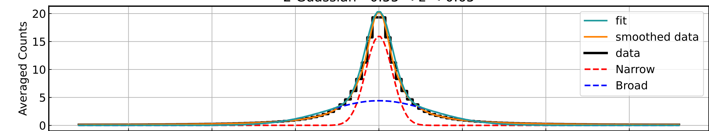
2 Guassian - 0.55 < z < 0.65
