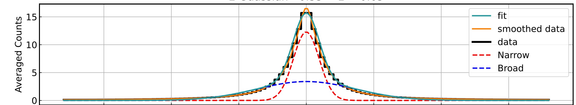
2 Guassian - 0.55 < z < 0.65
