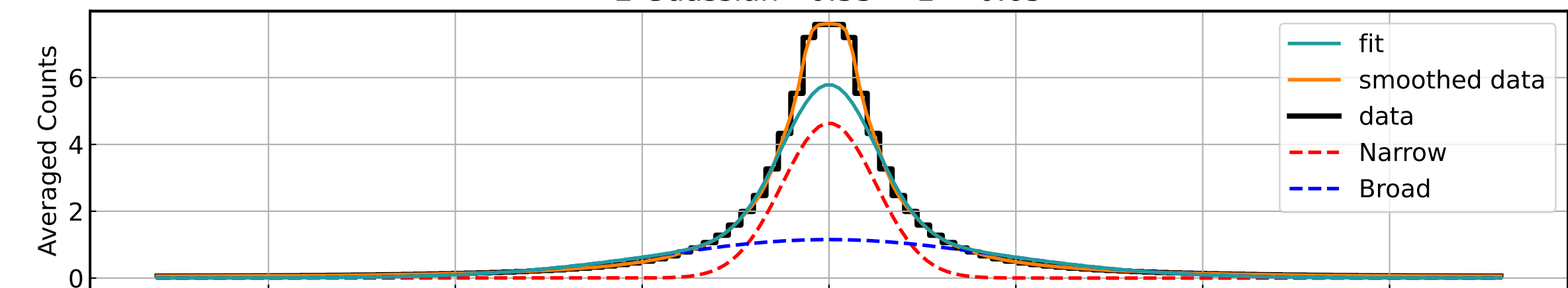
2 Guassian - 0.55 < z < 0.65
