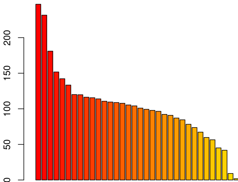
PCA eigenvalues
