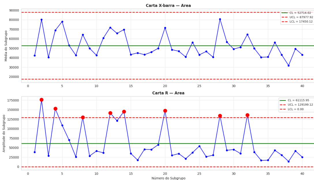
Gráfico 5. Cartas X-barra e R para Area. A média também é estável, mas oito subgrupos (20% da amostra) apresentam amplitude fora dos limites — sinal claro de causas especiais.
