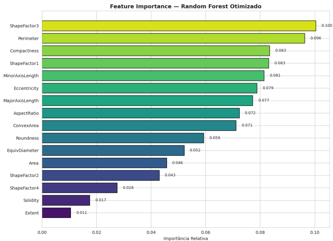
Gráfico 9. Importância das 16 features segundo o Random Forest otimizado. Shape factors e medidas de compactação aparecem entre as mais discriminantes.
