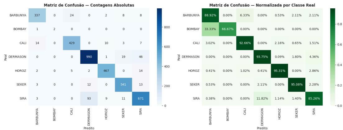
Gráfico 8. Matriz de confusão no conjunto de teste. A diagonal concentra a vasta maioria dos casos; a confusão mais relevante ocorre entre SIRA e DERMASON, variedades morfológicamente próximas.
