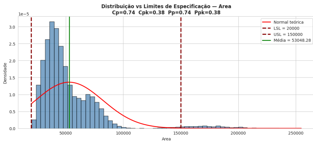
Gráfico 6. Distribuição de Área com indicação dos limites LSL e USL adotados. A cauda à direita (BOMBAY) puxa a média para longe do centro do intervalo de especificação, gerando Cpk = 0,38 .
