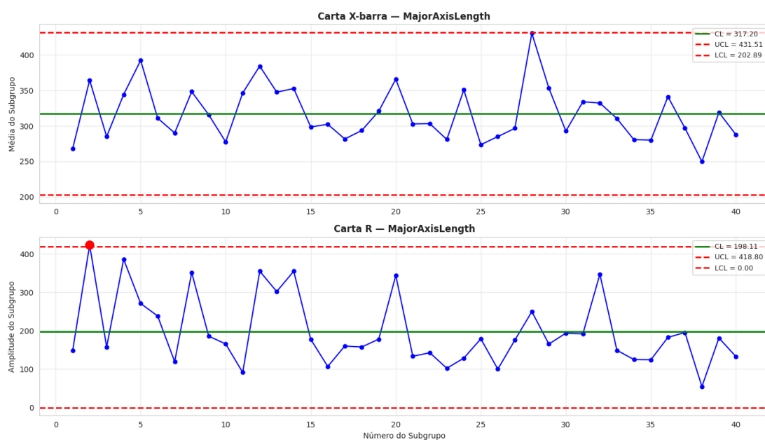
Gráfico 4. Cartas X-barra e R para MajorAxisLength, com n=5 e 40 subgrupos. A média permanece estável dentro dos limites, mas a amplitude apresenta um ponto isolado acima do UCL.
