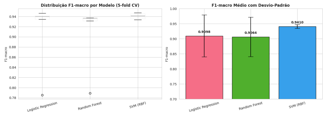
Gráfico 7. Comparação dos três modelos por validação cruzada. As caixas indicam dispersão entre os cinco folds — o SVM destaca-se não tanto pela média superior, mas pela consistência (caixa quase imperceptível).
