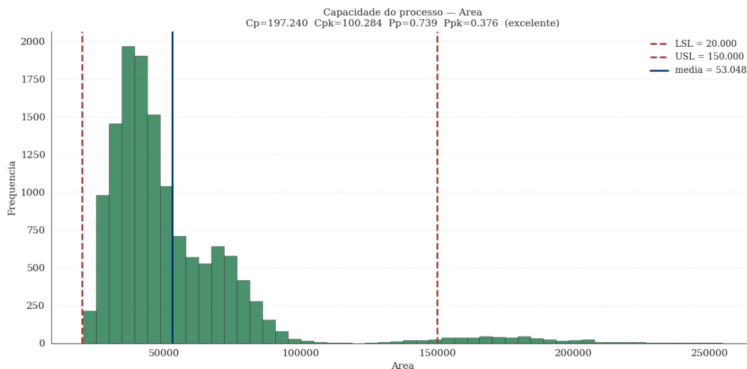
Gráfico 6. Distribuição de Área com indicação dos limites LSL e USL adotados. A cauda à direita (BOMBAY) puxa a média para longe do centro do intervalo de especificação, gerando Ppk = 0,38 .
