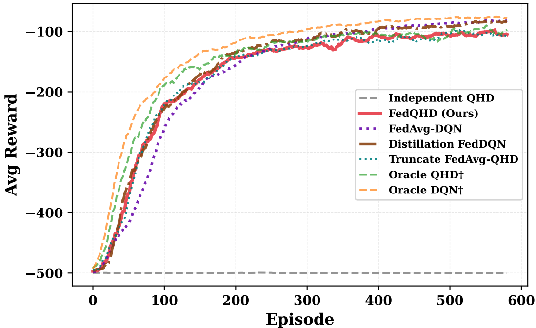
Acrobot-v1 — Q1: Homogeneous Encoders
