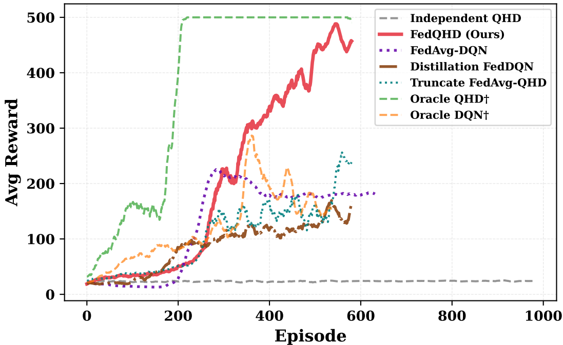
CartPole-v1 — Q1: Homogeneous Encoders
