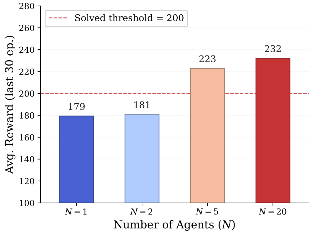
LunarLander-v3
