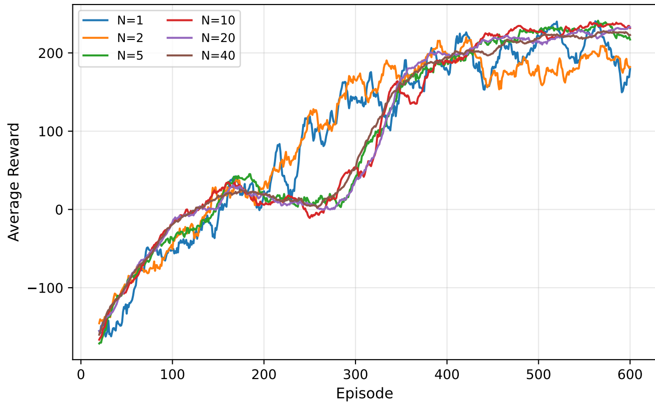
FedQHD
