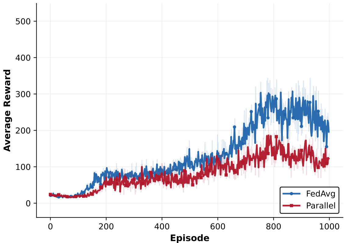
DQN
