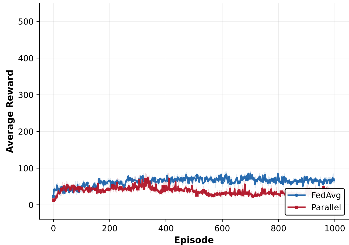
Linear SARSA
