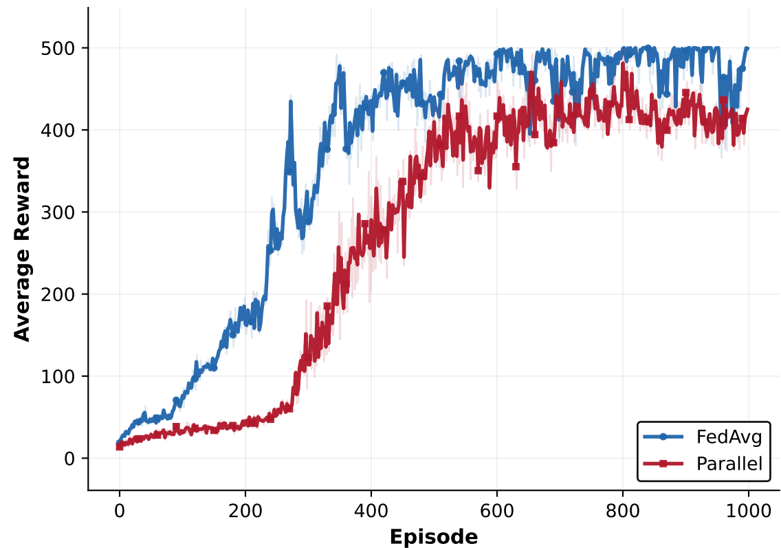
HD SARSA
