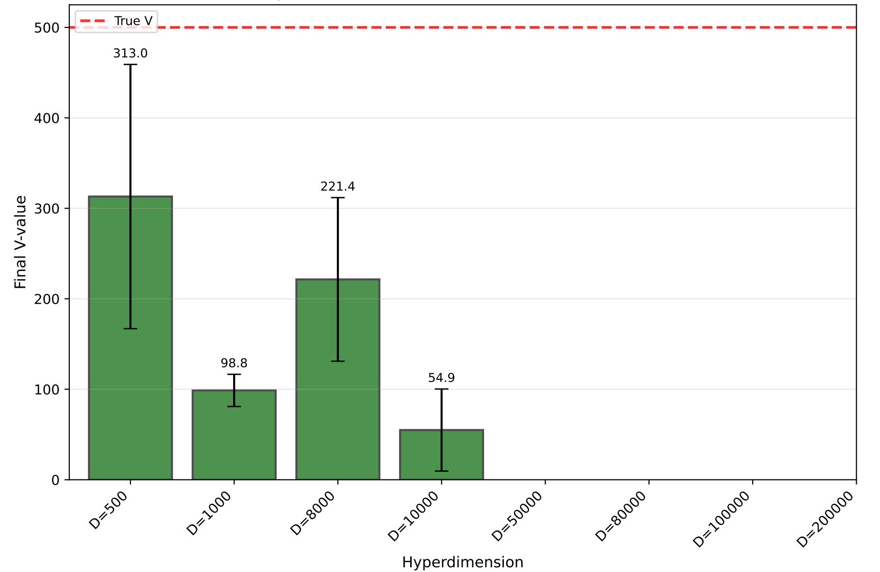
(d) Hyperdimension Ablation: Final V-values (N=2)
